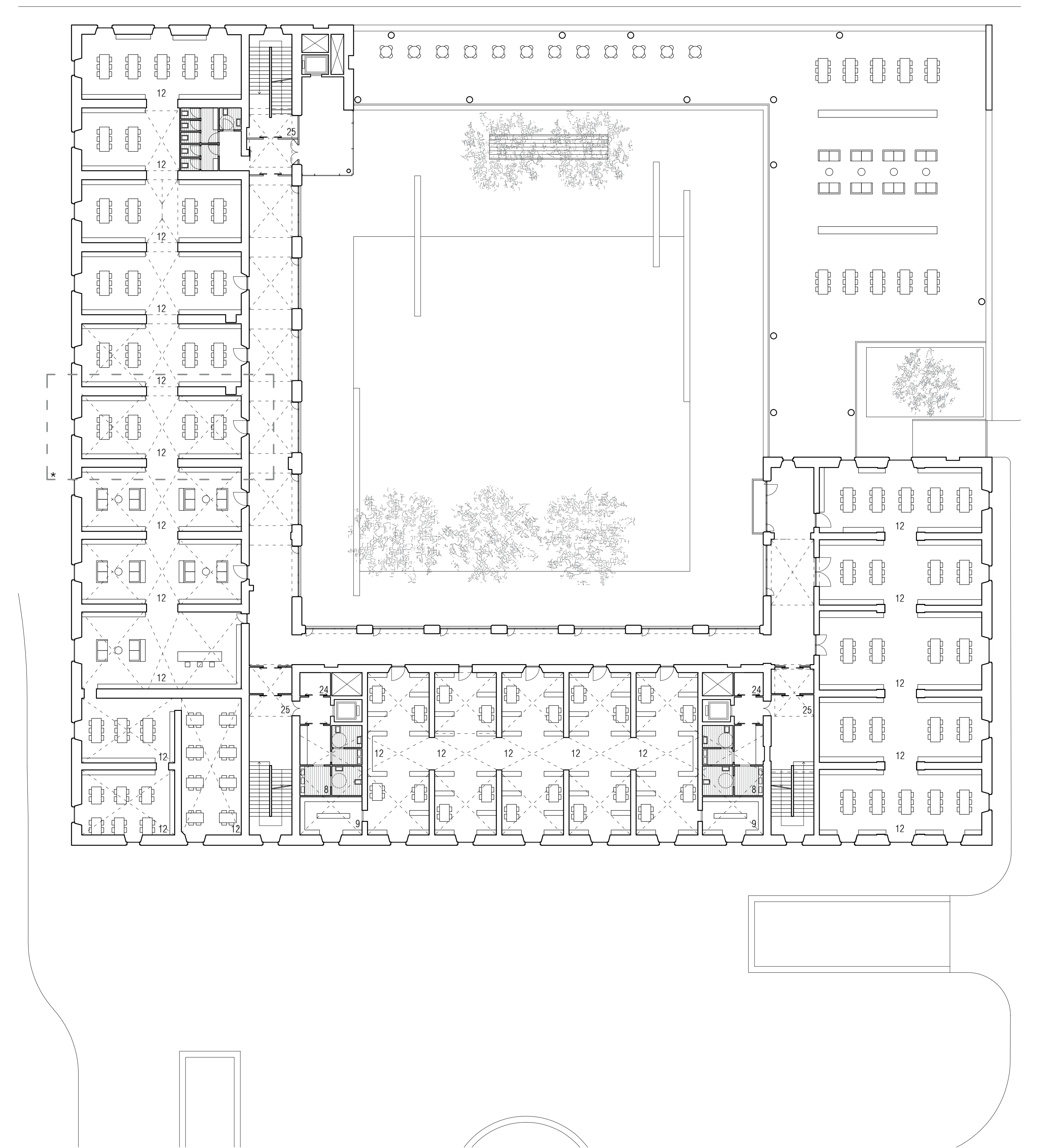
PIANTA PIANO SECONDO
