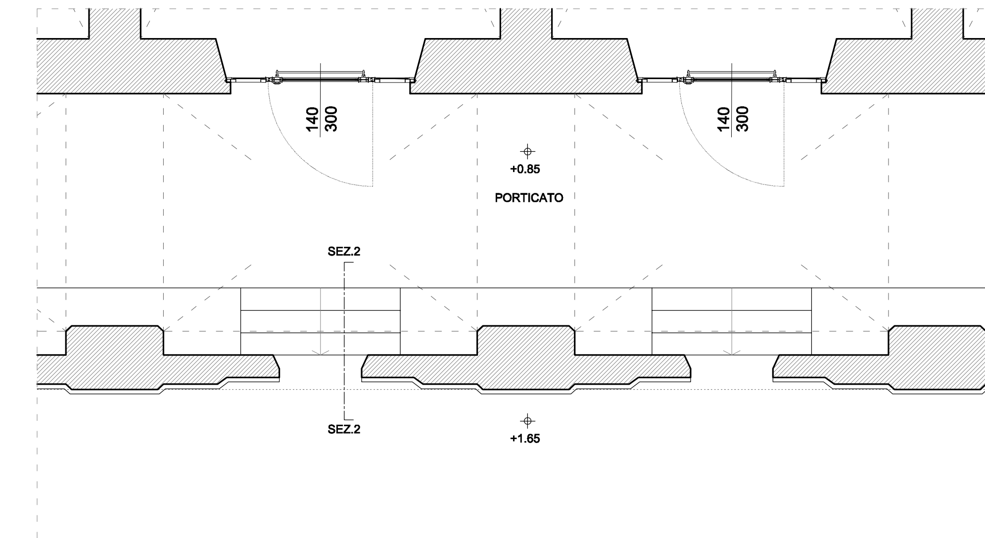
Pianta di progetto _ scala 1:50
