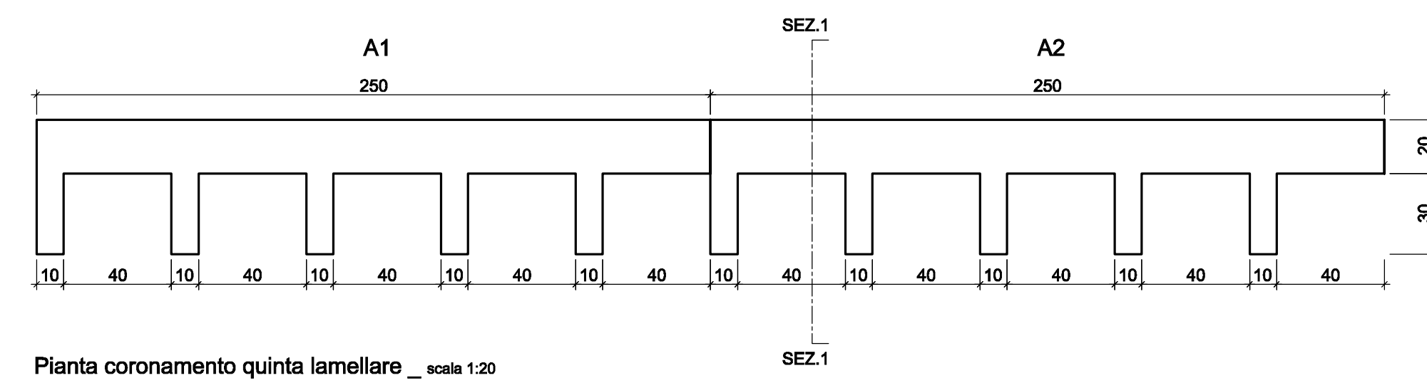
Pianta coronamento quinta lamellare _ scala 1:20
