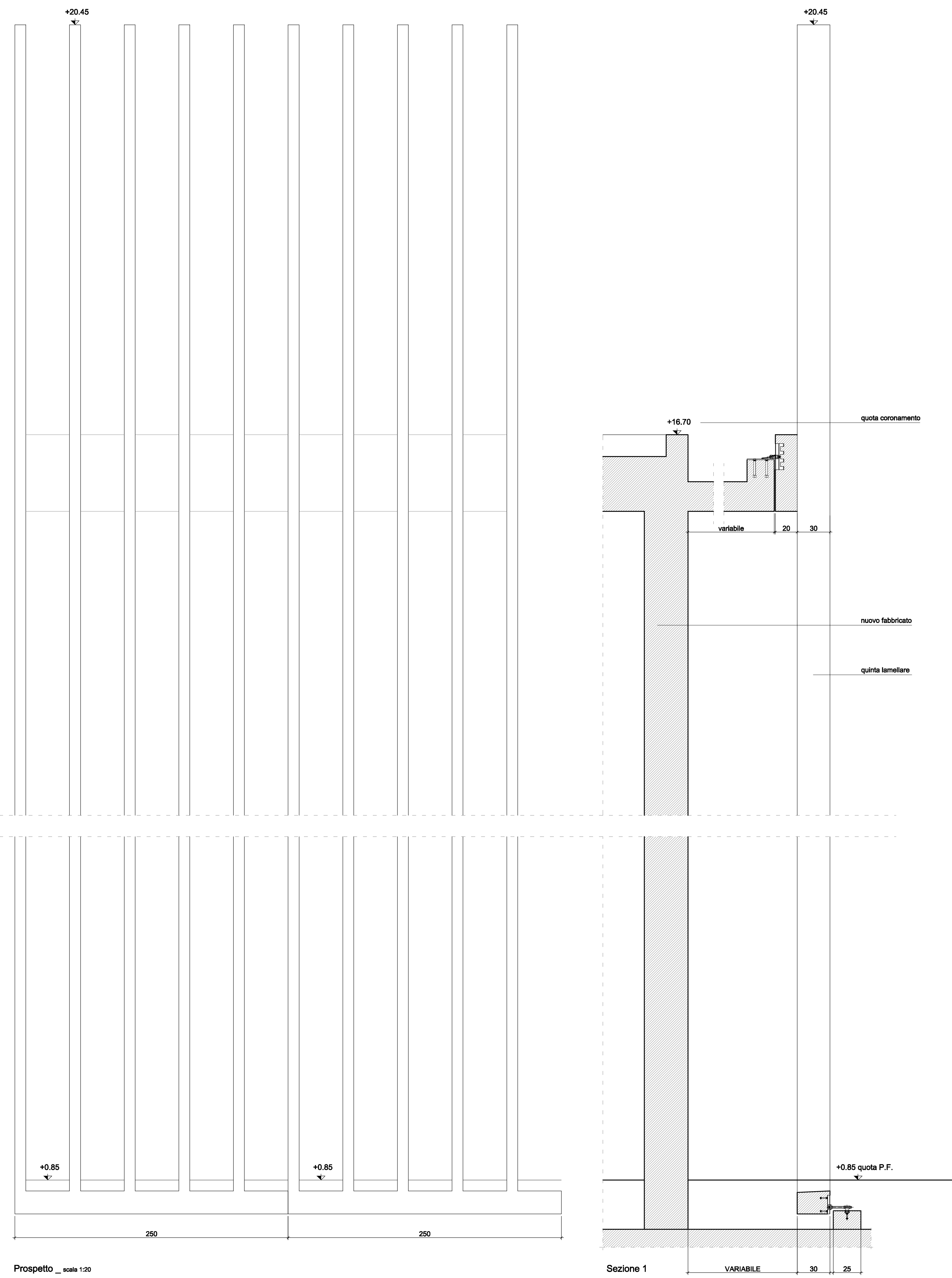
Prospetto _ scala 1:20
