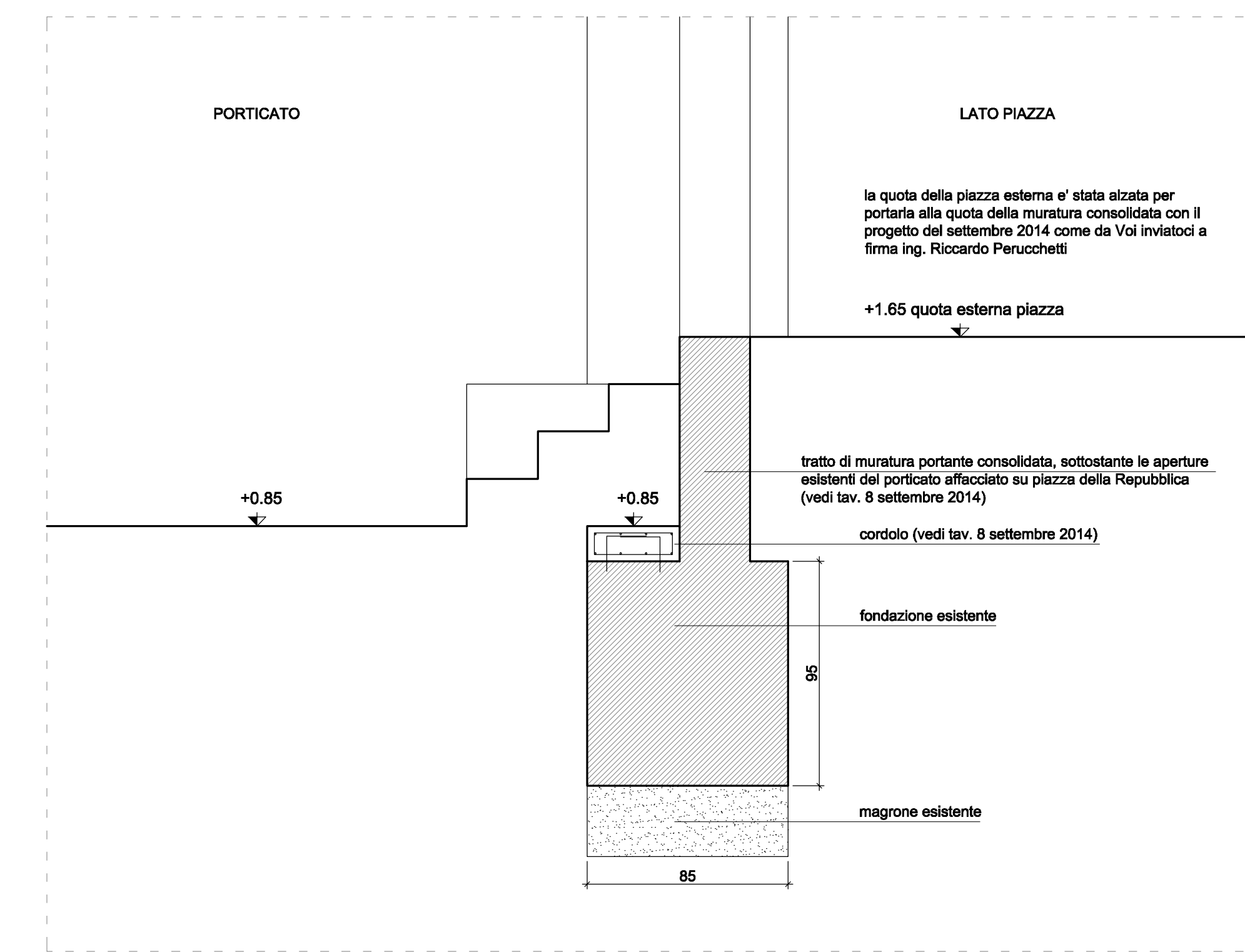
Sezione 2 _ scala 1:20
