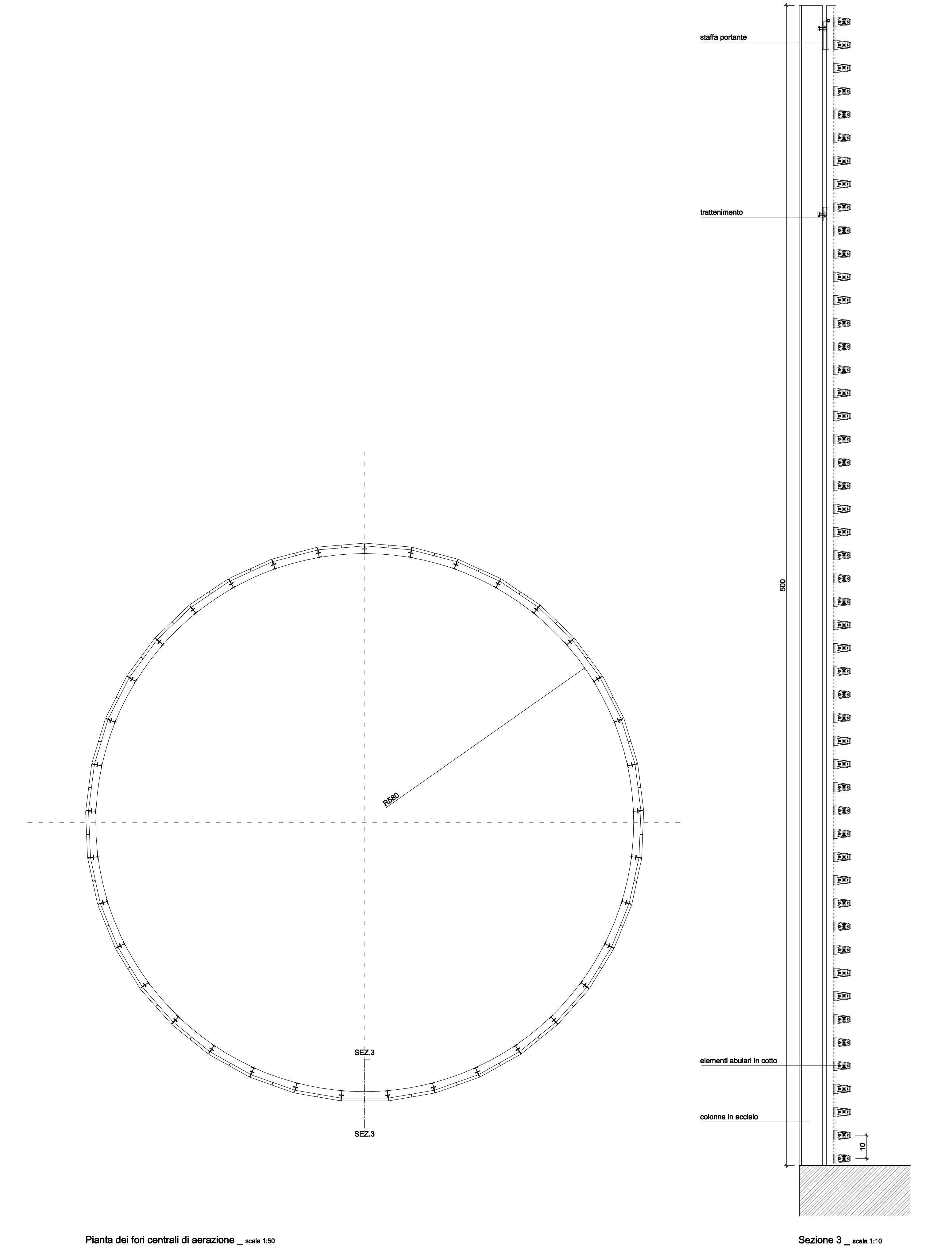
Pianta dei fori centrali di aerazione _ scala 1:50
