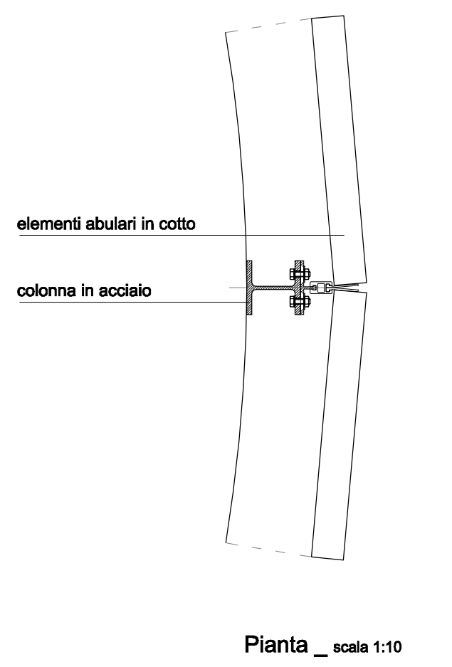
Pianta _ scala 1:10
