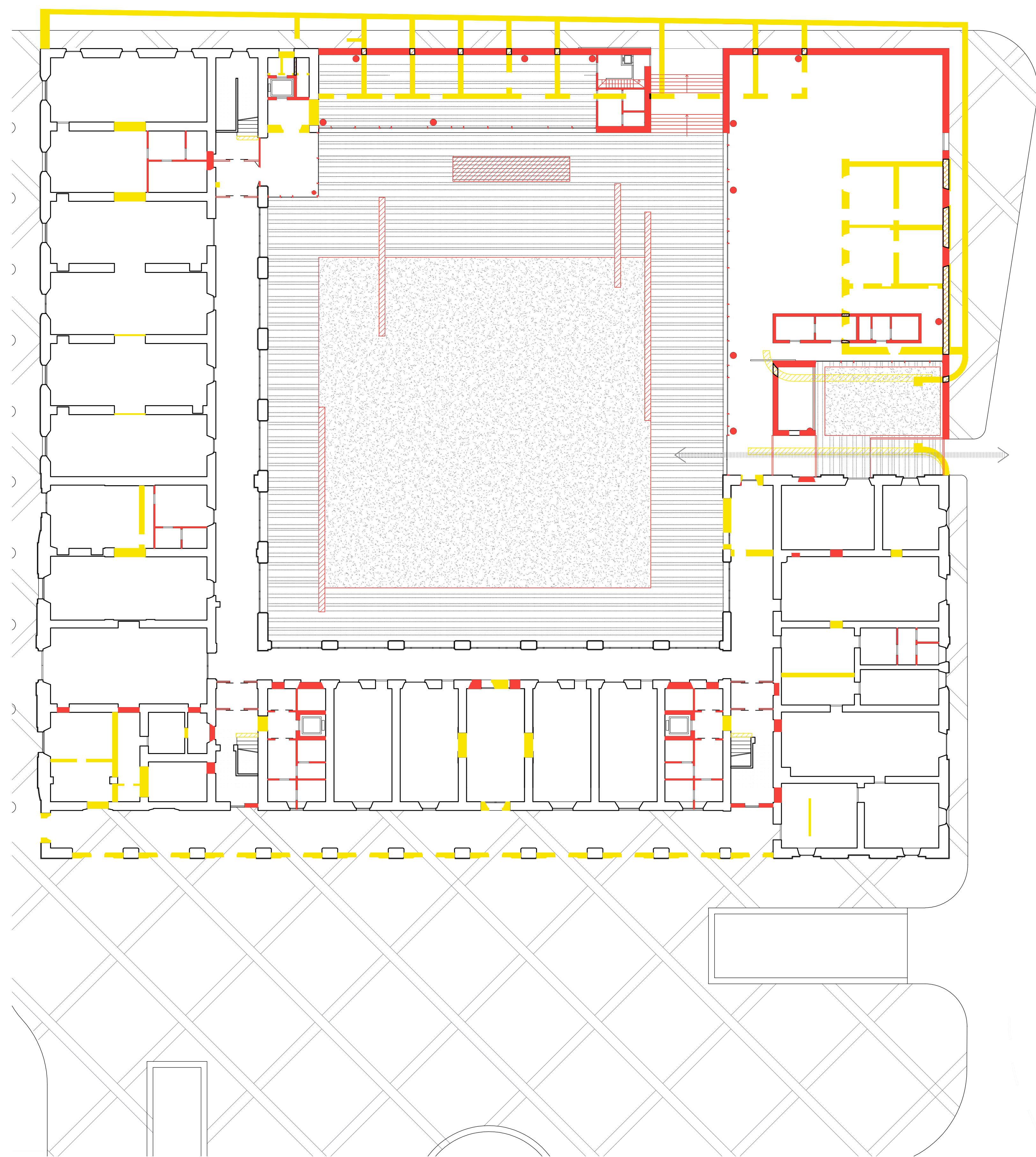
COMPARATO PIANTA PIANO TERRA
